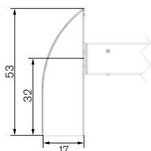
CONTURA POUR BASSIN JUSQU'À 5 M DE LARGE.
